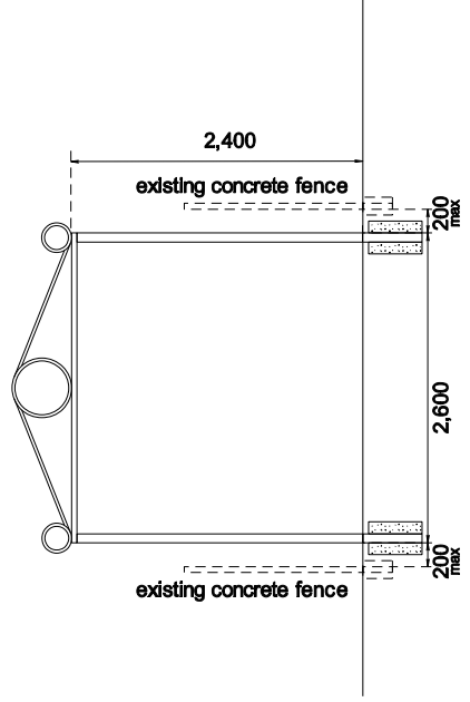
TPK29 - Elevation 1:50
