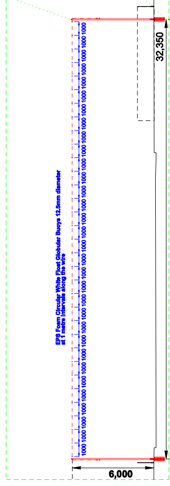
TP28 - Elevation
