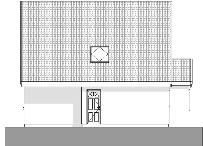
E2 | Left Elevation (Existing) 1:50
